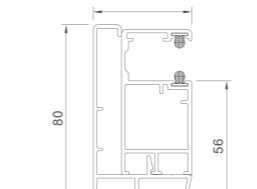
Einseitige Führungsschiene (ALU) - RSZ A973+A933
