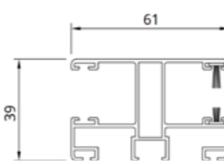
Einseitige / Doppel Führungsschiene (ALU) 01130903BL
