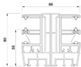
Doppel Führungsschiene (PVC) + INS* - RS Revision von außen. MK8120 + MK9730
