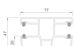
Zweiseitige Führungsschiene (ALU) - RSW A939
